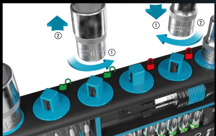
Im geschlossenen Zustand sind alle Teile stets sicher arretiert. Ein Herausfallen ist unmöglich! Zur Entnahme Steckschlüsseinsatz drehen und nach oben abziehen
